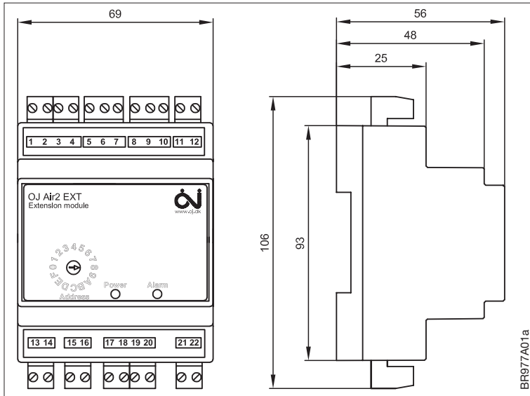
Fig. 1 - Dimensions
