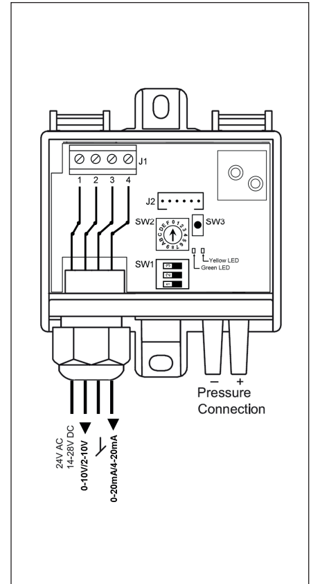
Fig. 3 - Wiring diagram
