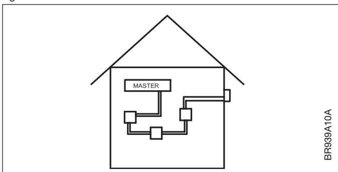
Føler og utekompenseringsenhet koblet i bussmodus (kjedekoblet)
