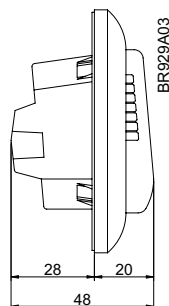
Abmessungen (mm)
