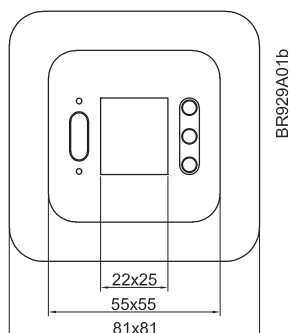
Abmessungen (mm)
